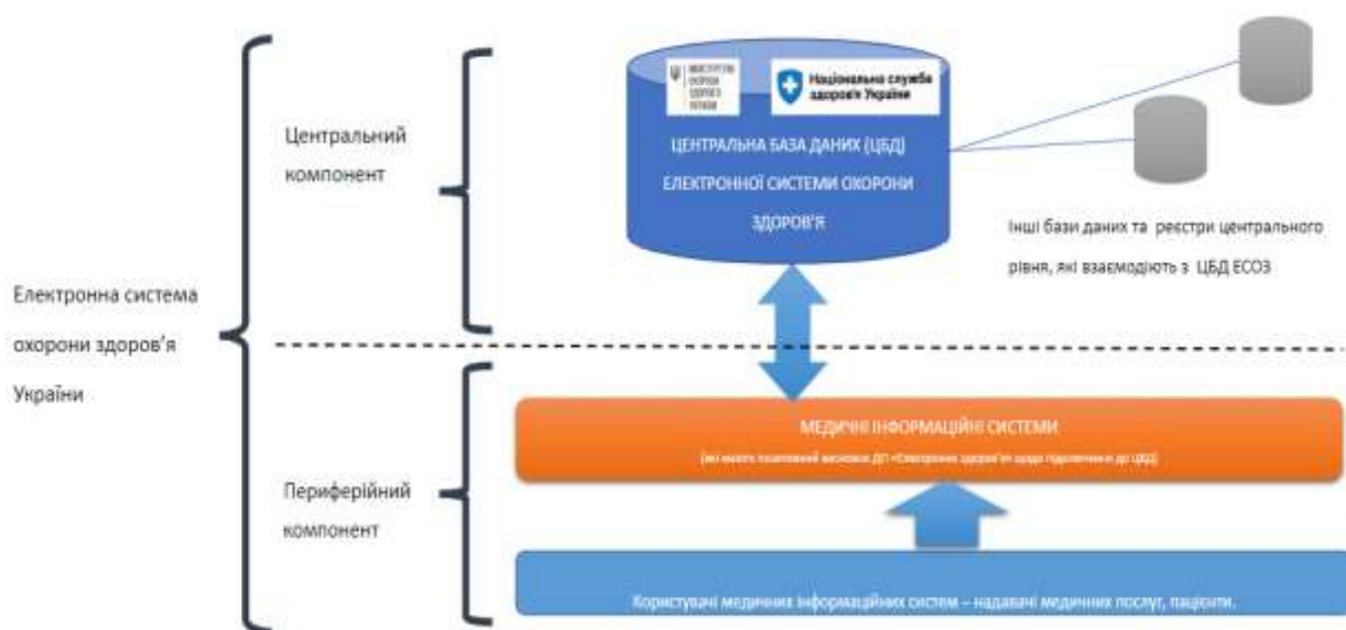
Рисунок 1. Архітектура ЕСОЗ
